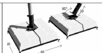
Base para maxi sombrillas
