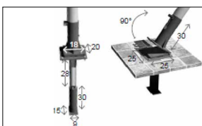
Base con tubo para conexión
